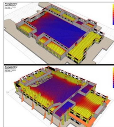
Gambar 4. Simulasi pencahayaan alami [21]
