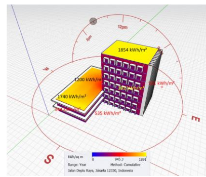
Gambar 3. Modeling dan simulasi radiasi panas matahari dengan Formit
